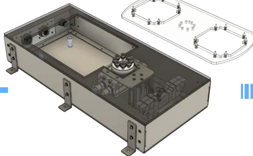
2ポジションターンテーブル
