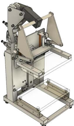
自動式プレスユニット
